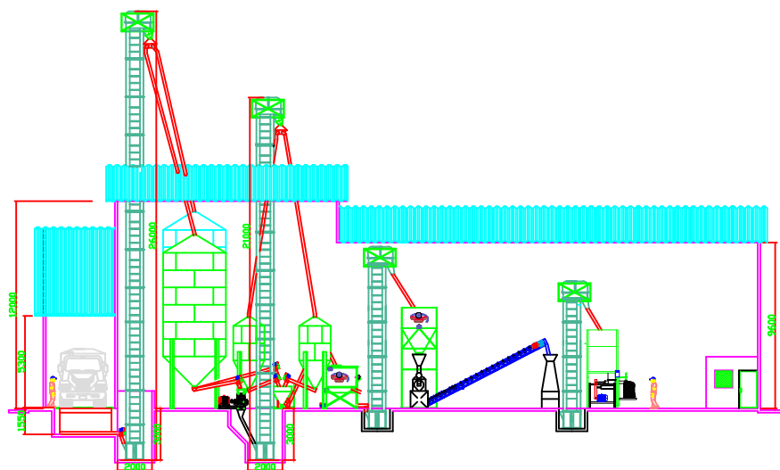
CORTE A-A
