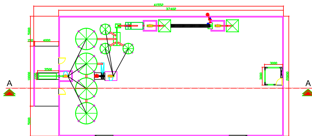
PLANTA BAIXA
